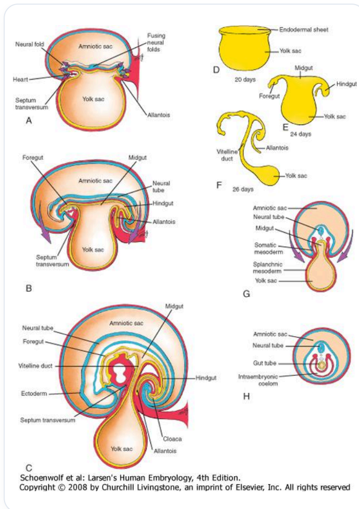
ABB. — Entwicklung des embryonalen Verdauungstrakts
